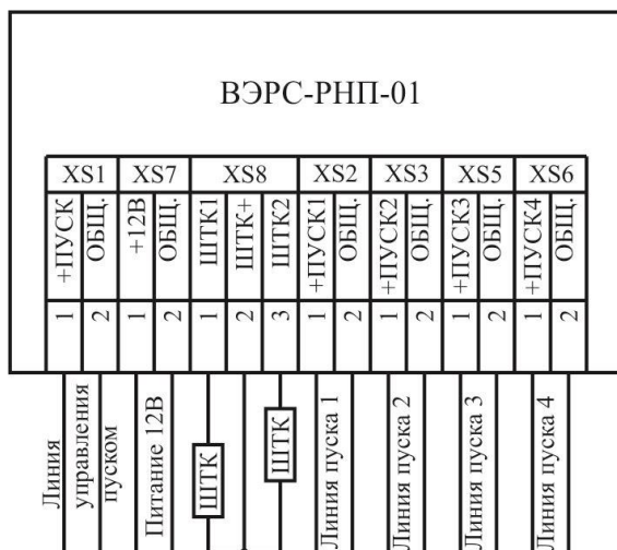
Рис. 3. Схема внешних соединений.
